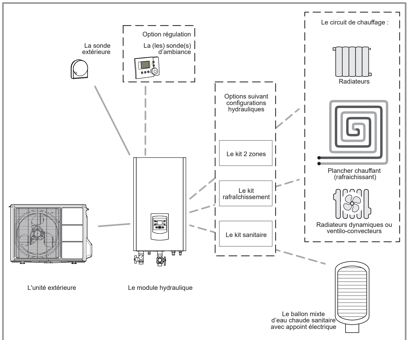
figure 1 - Vue d'ensemble d'une configuration d'installation complète
