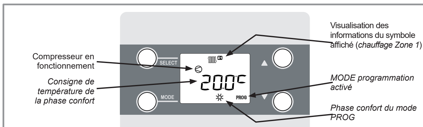
figure 4 - Interface utilisateur (exemple d'affichage de base)
