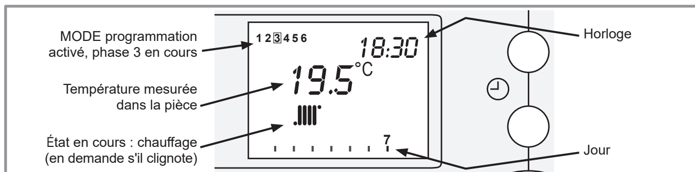
figure 6 - Sonde d'ambiance (exemple d'affichage de base)
