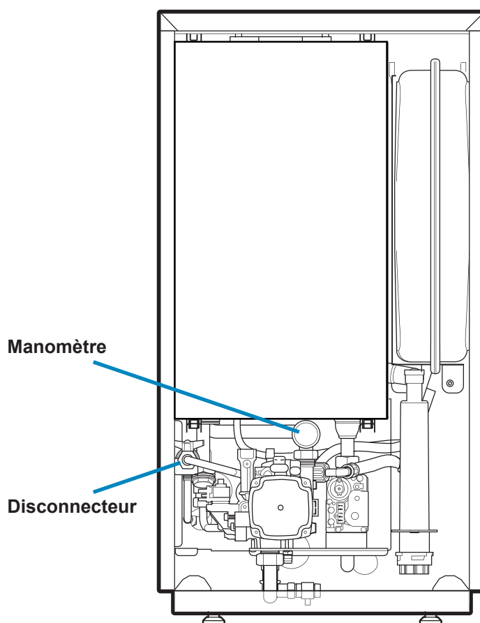
fig. 5 - Perfinox 2 - Emplacement du disconnecteur
