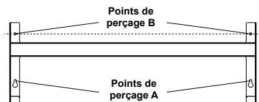
Modèle Plinthe
