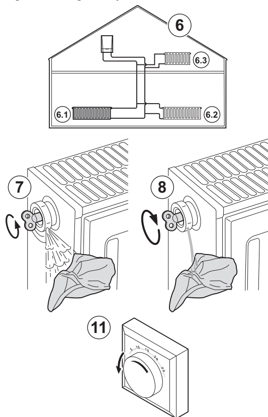
Fig.33 Purge du système
