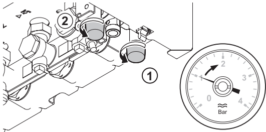
Fig.29 Ouvrir les robinets du disconnecteur
