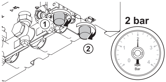
Fig.30 Refermer les robinets du disconnecteur
