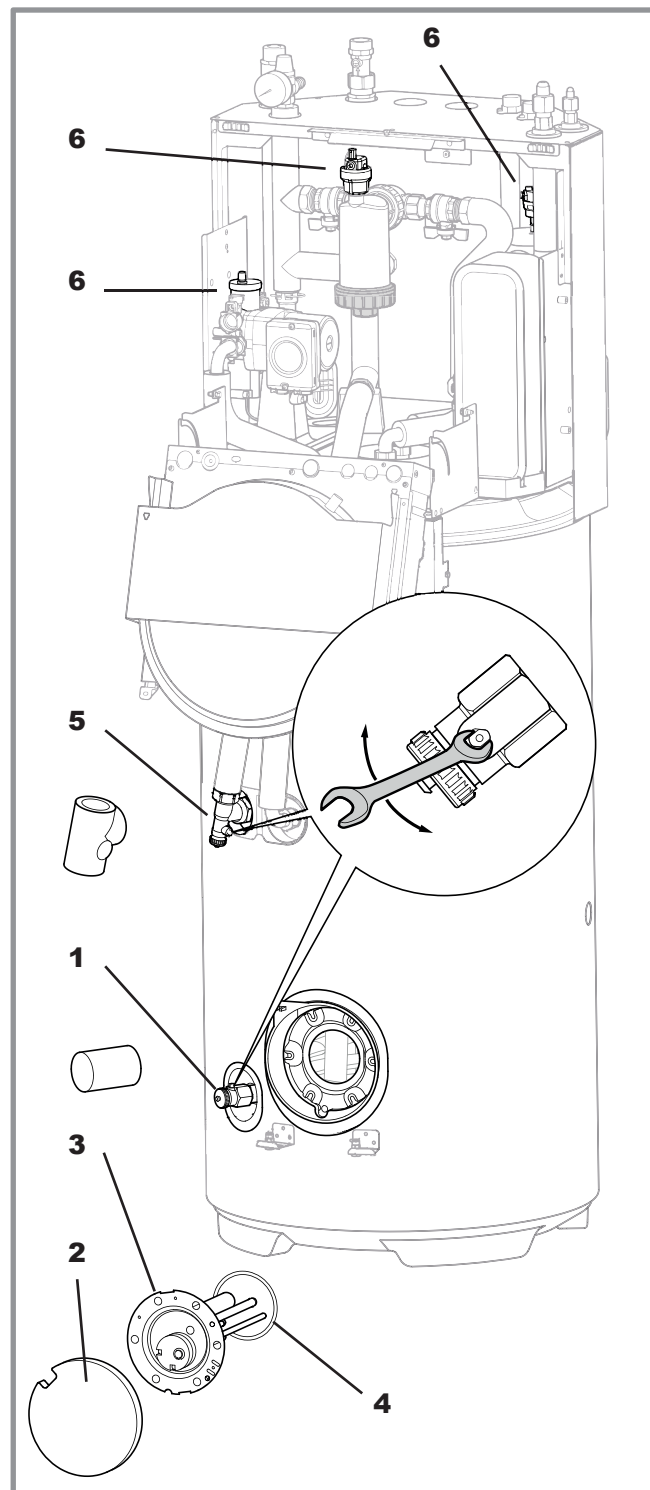
figure 43 - Vidange du module hydraulique et/ou du ballon sanitaire
