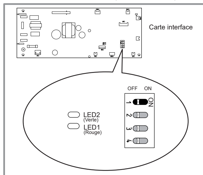
figure 20 - Emplacement des interrupteurs DIP et des LED sur la carte d'interface du module hydraulique
