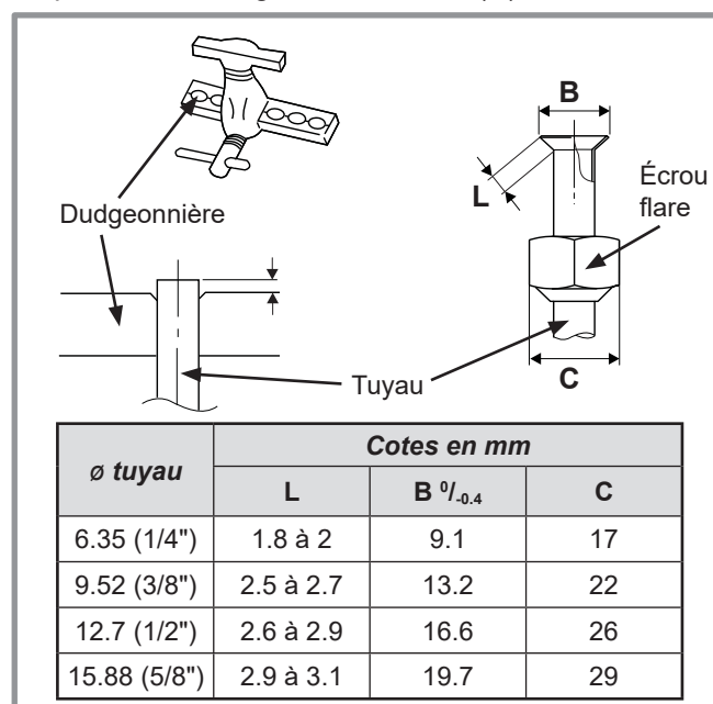
figure 14 - Évasement pour liaisons flare
