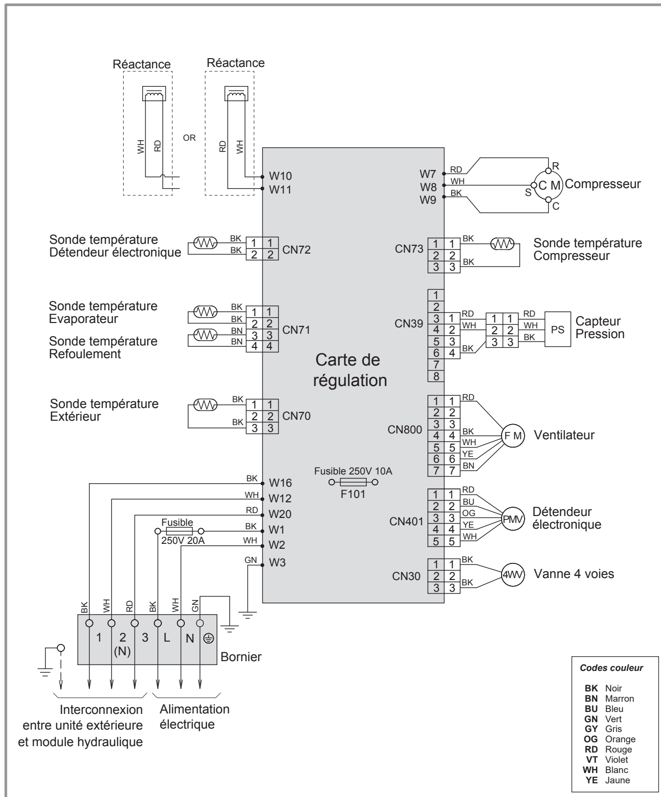
figure 46 - Câblage électrique unité extérieure Modèle Loria duo 6004 & 6006
