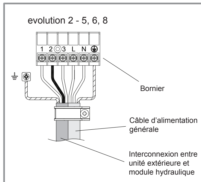
figure 26 - Connexions au bornier de l'unité extérieure
