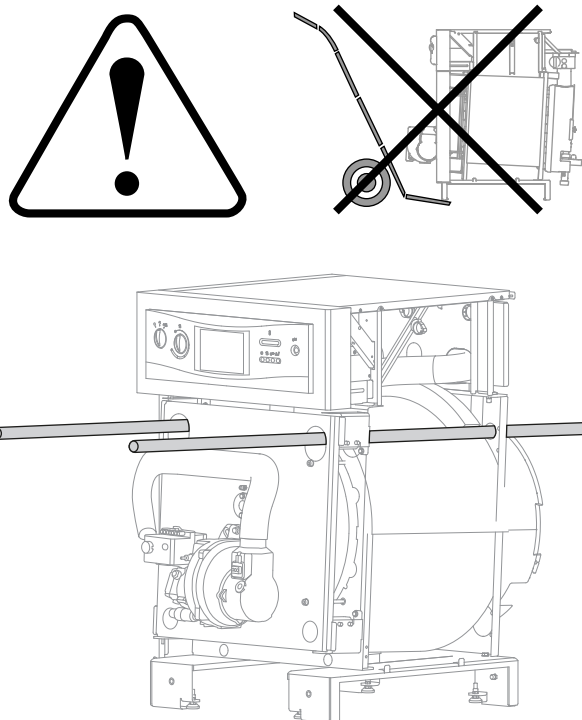
fig. 11 - Transport et levage de la chaudière
