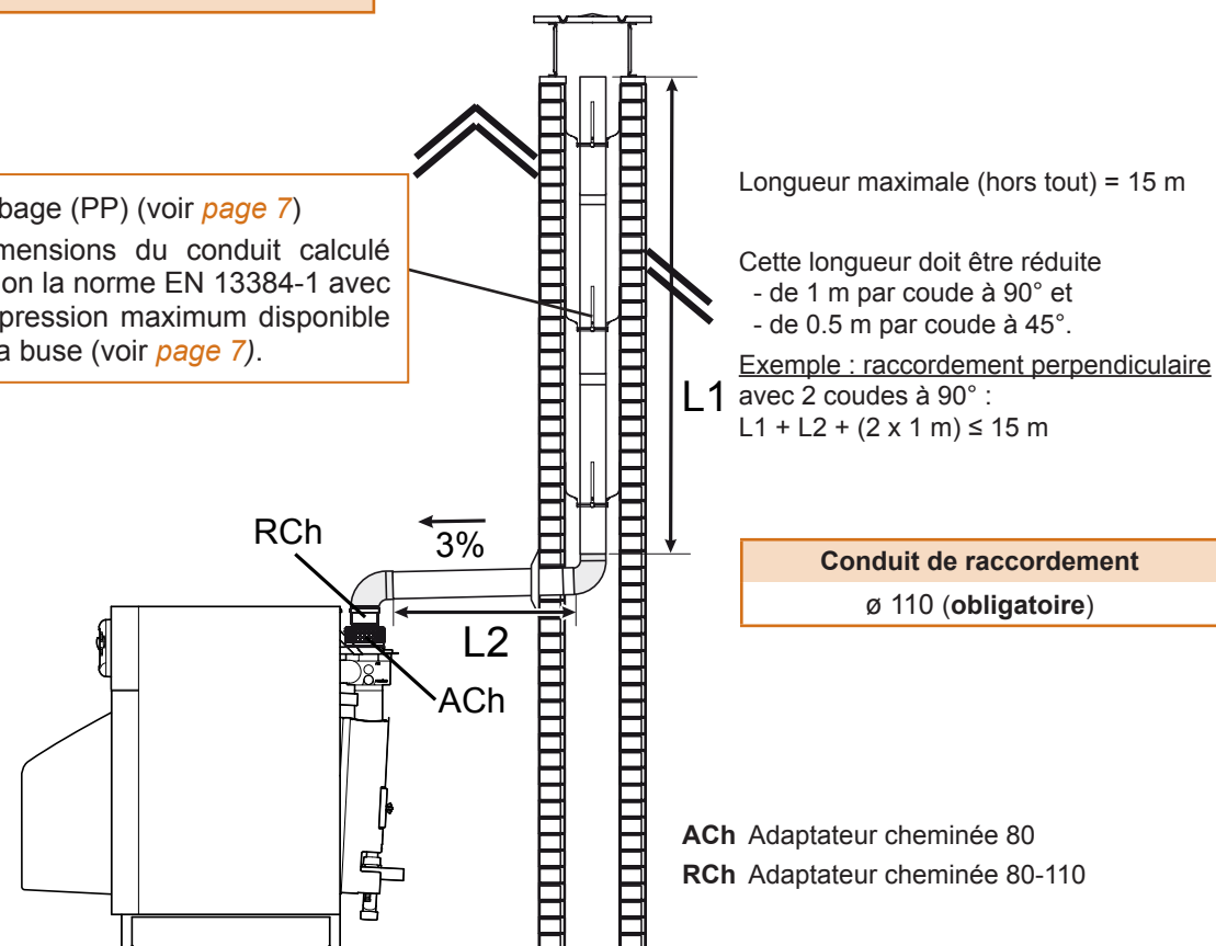
fig. 15 - Possibilités de raccordement (type B23 et B23P)
