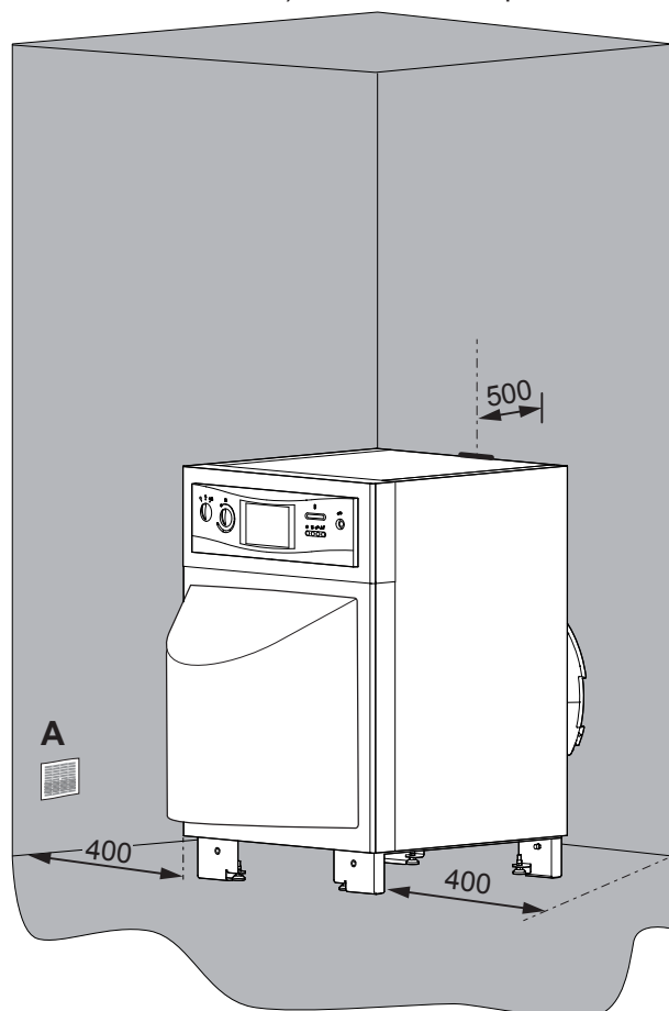
fig. 10 - Dégagements minimum d'installation autour de la chaudière
