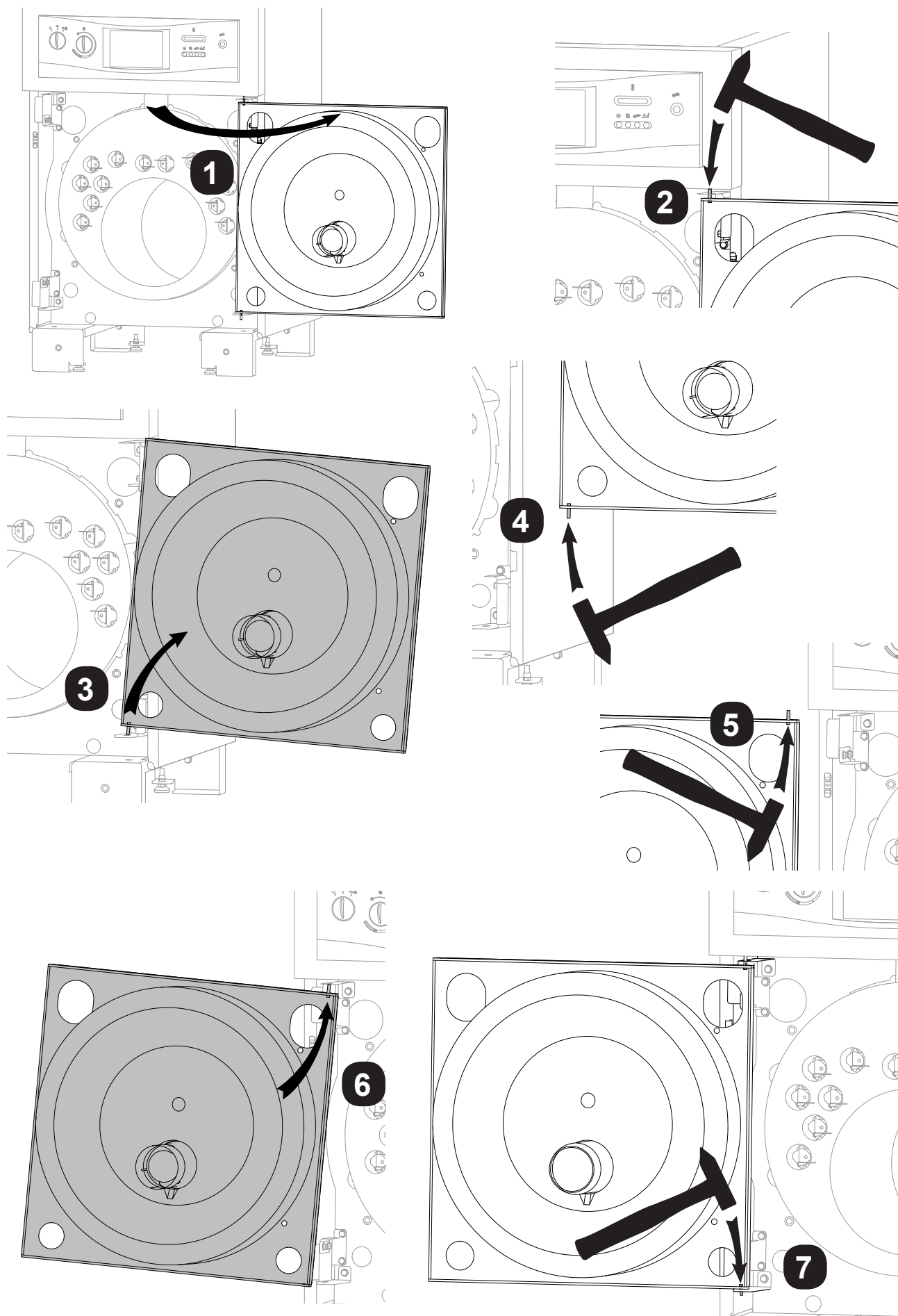
fig. 6 - Changement de sens d'ouverture de la porte foyer
