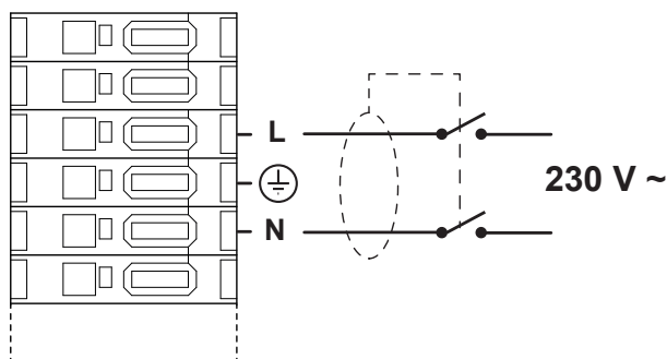
fig. 21 - Protection différentielle
