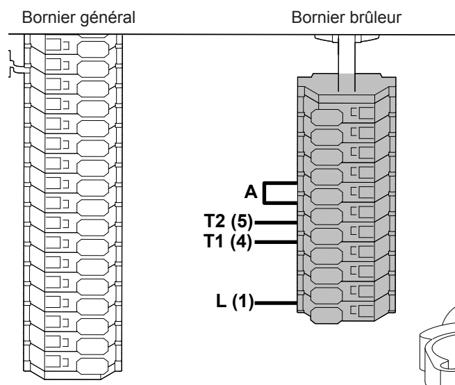
fig. 29 - Bornier brûleur
