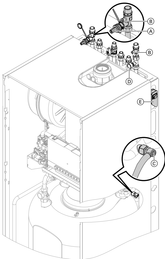
Fig. 26 Illustration avec les raccordements vers le haut
