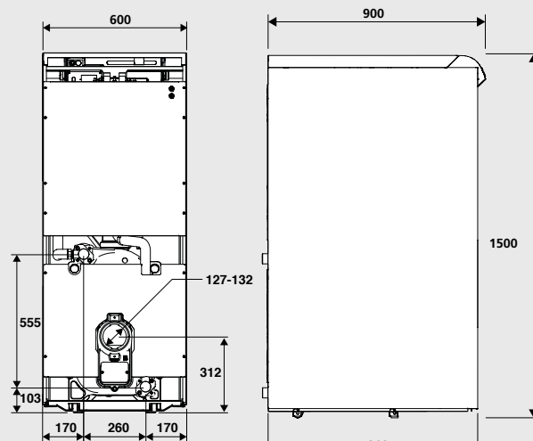
Vue arrière
