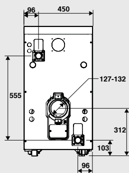
Vue arrière
