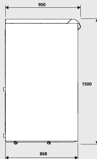
Vue côté
