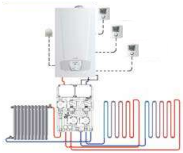
Luna Platinum + HTE avec module partage + 3 zones
